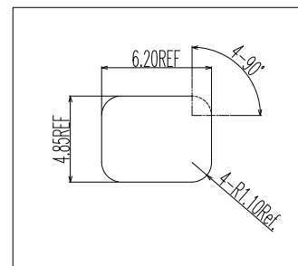
面板开孔参考尺寸
