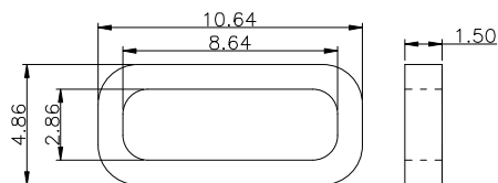
建议的胶圈尺寸
