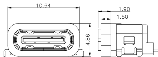
加防水圈示意图
