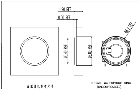
面板开孔参考尺寸
