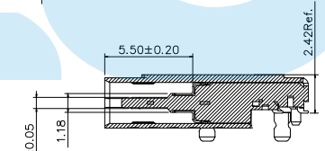
剖面图 比例: 1 A-A
